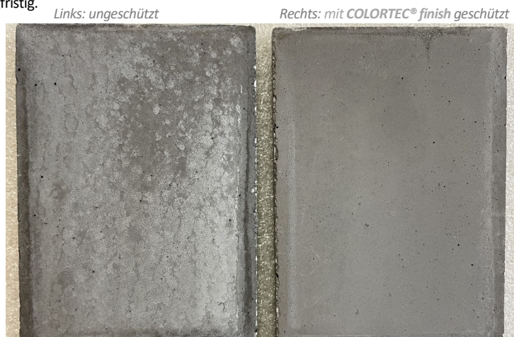
Foto nach längerer Bewitterung der Betonoberfläche im Freien.
